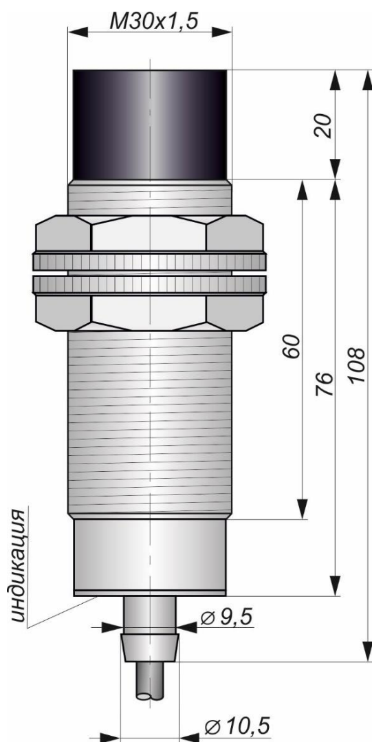
Габаритный чертеж
